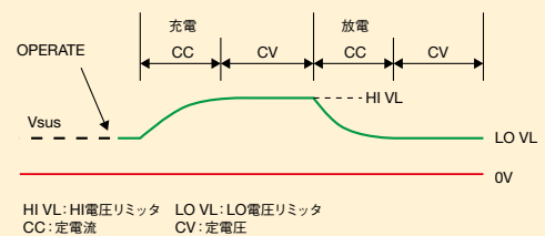
バッテリー充電波形
