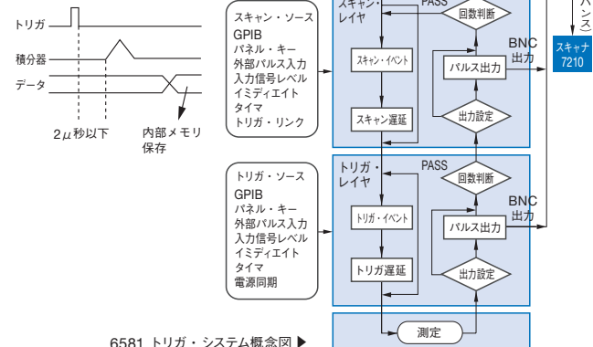
6581 トリガ・システム概念図
