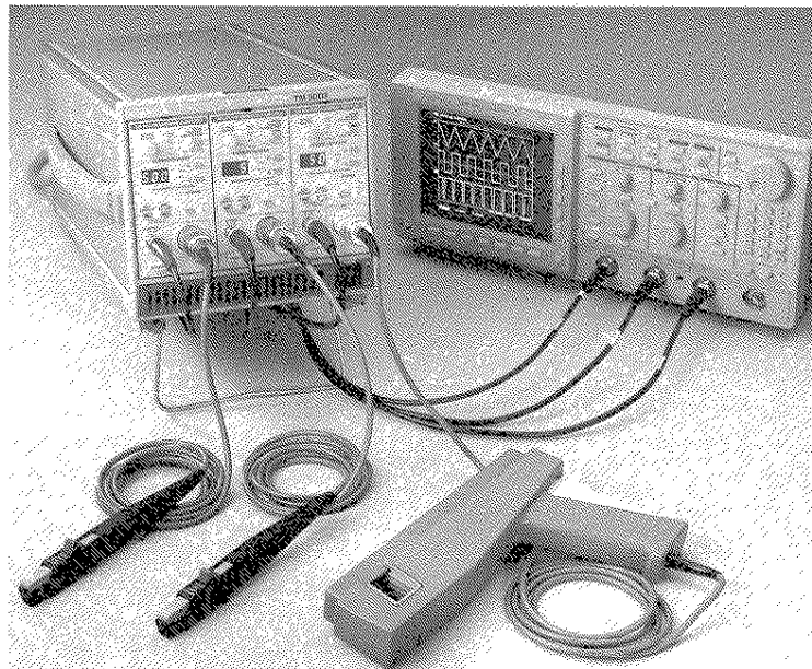
AM5030型/TM5003型メイン・フレーム組込み例(左上)、A6302型(左下)およびA6303型(右下)電流プローブ
