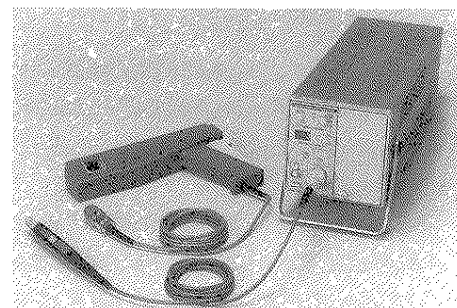
AM503B型/TM502Aオプション13型組合せ(右)、A6303型(左上)およびA6302型(左下)電流プローブ
