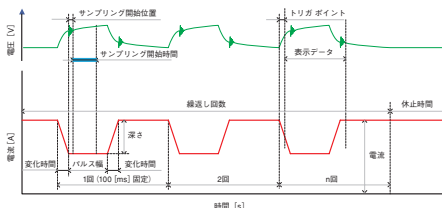
▲電流遮断測定
