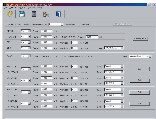
HSDPA IQproducer の設定画面例
