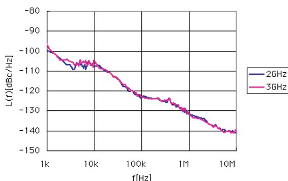
SSB位相雑音の一例( 2.5 MHz < f < 3 GHz ) ( CW、コンティニュアスモード：OFF、周波数切替スピード：ノーマル )
