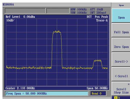
出力波形
