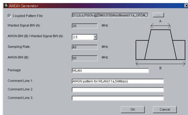
AWGN画面例
