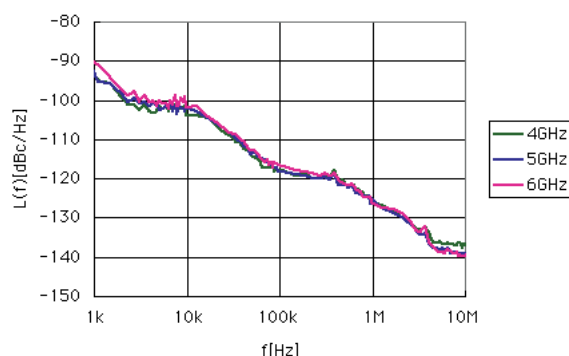
SSB位相雑音の一例( 3 GHz < f < 6 GHz ) ( CW、コンティニュアスモード：OFF、周波数切替スピード：ノーマル )
