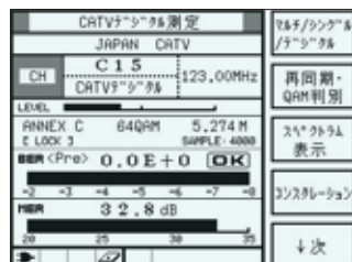
BER と MER 測定 (CATVデジタル)
