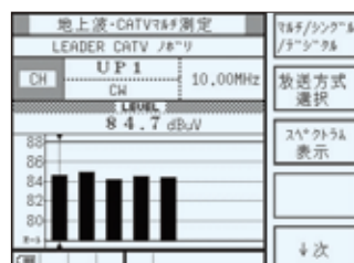
CATV 上り回線測定
