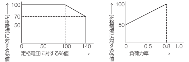
図2 許容負荷力率
