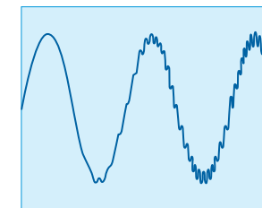
中間高調波の重畳 (サブシンセサイザV/Fスイープ)
