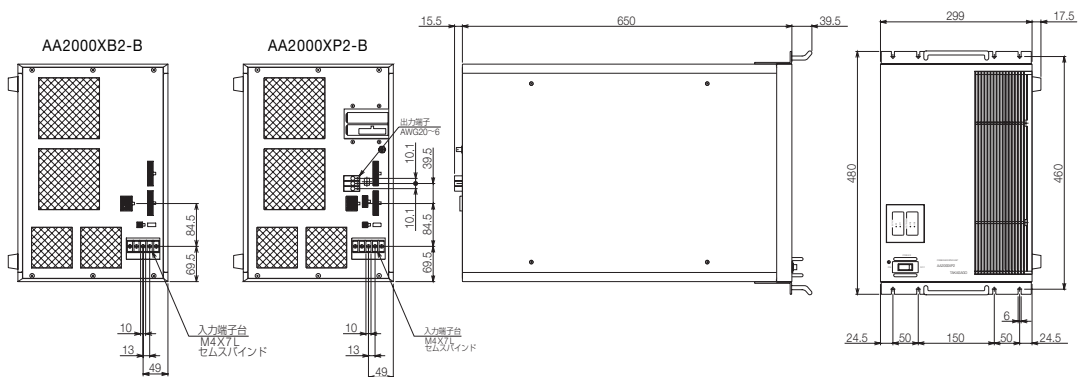
AA2000XB2-B AA2000XP2-B
