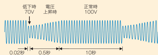
電圧変化のシミュレーション例
