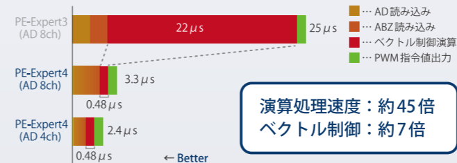
当社モータコントロールSW使用時の処理速度比較 (2014.8.22)
