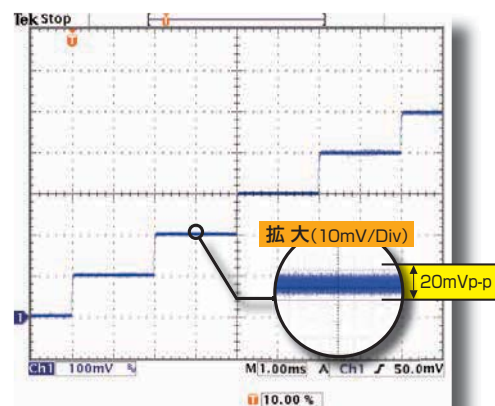
▲ 0.1V ステップ実波形サンプル
