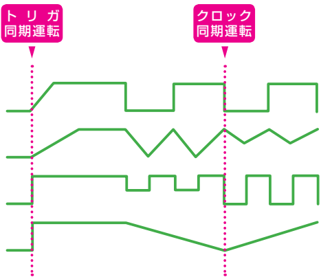
▲トリガ、クロック併用同期運転例
