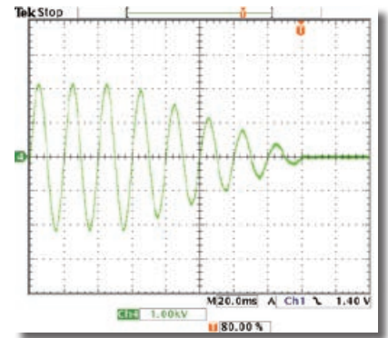
▲フォールタイム制御波形例
