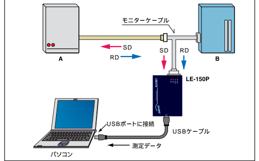
付属の解析ソフトをインストールしたUSBポートを持つパソコン
