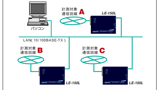
付属の解析ソフトをインストールした10/100Base-TXポートを装備したパソコン。解析ソフトから複数のアナライザーをコントロールする場合は、解析ソフトの設定画面でアナライザーのIPアドレスを指定して識別します。
