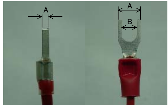
圧着端子形状
